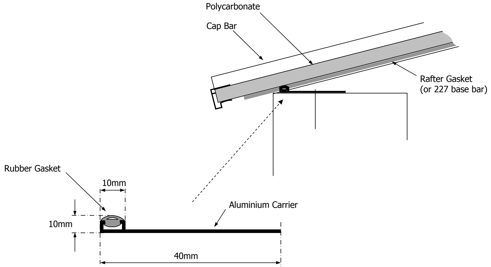
P226F Eaves Filler
